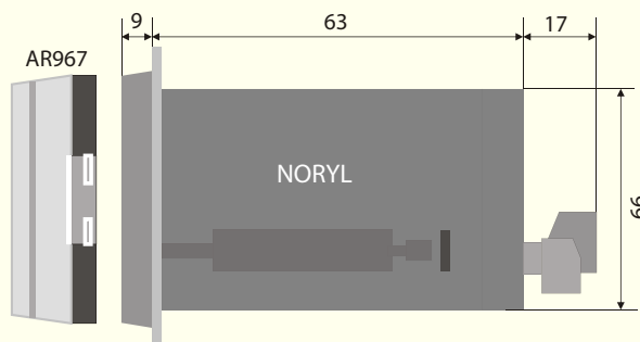
WIDOK OD STRONY UCHWYTU MOCUJĄCEGO
